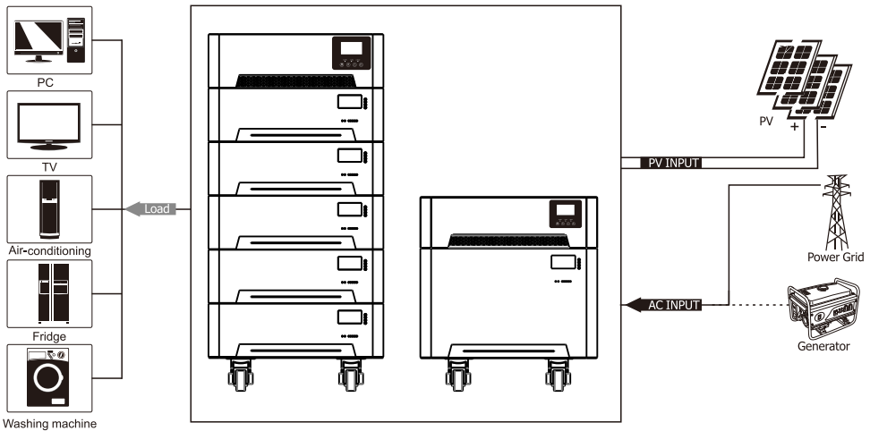
Рис. 1 Гібридна система електропостачання
