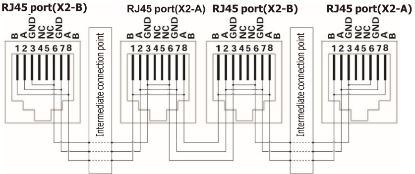
Схема з'єднання паралельних кабелів RS485
